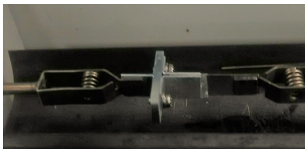
Fig.2 剪断治具をセットした状態
