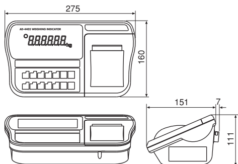
AD-4405 寸法図
