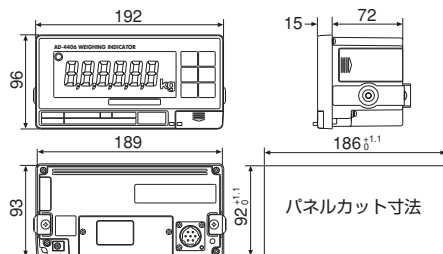
AD-4406 寸法図
